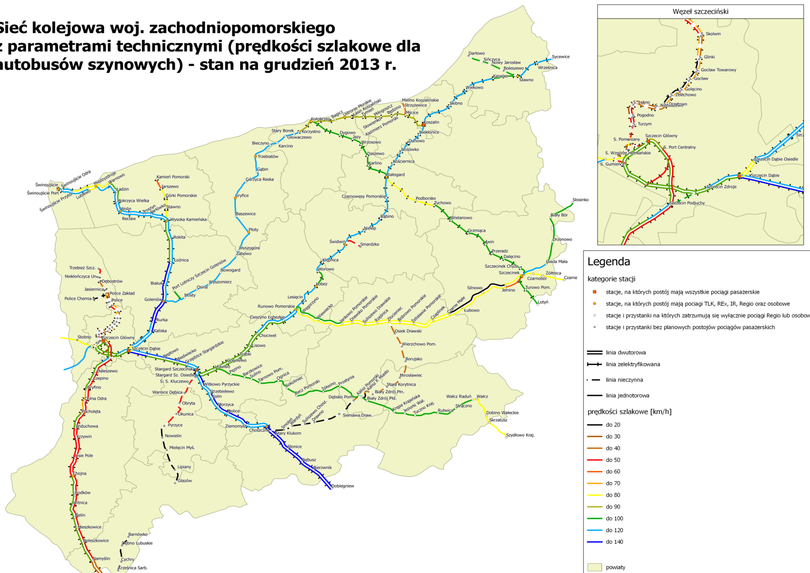
Rys. 4.1.2. Parametry techniczne (prędkości szlakowej dla autobusów szynowych) sieci kolejowej w województwie zachodniopomorskim – stan na grudzień 2013 r.
