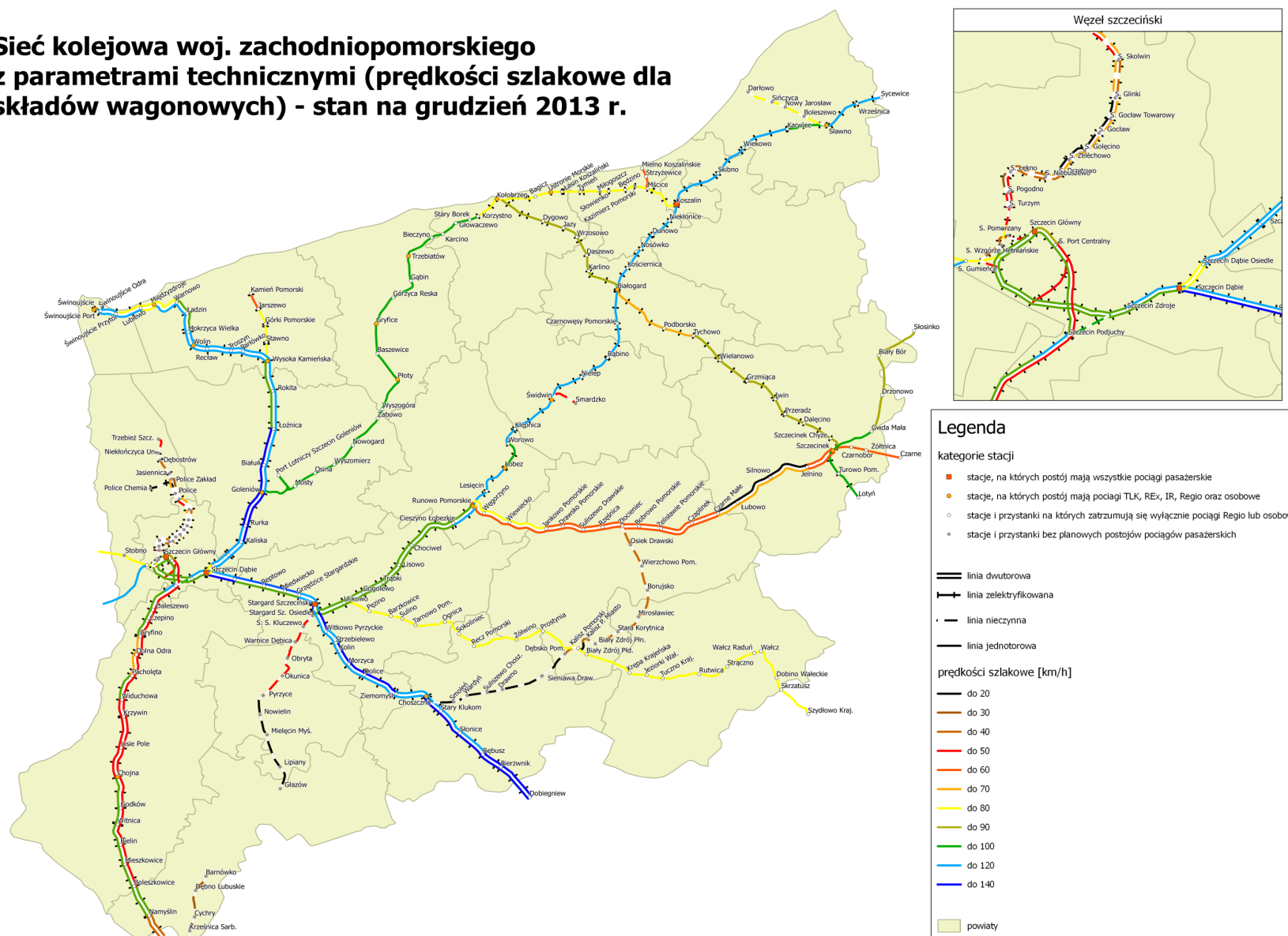
Rys. 4.1.3. Parametry techniczne (prędkości szlakowej dla składów wagonowych) sieci kolejowej w województwie zachodniopomorskim – stan na grudzień 2013 r.
